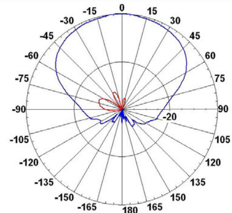
5.5 Ghz H-Plane and E of H-Plane
